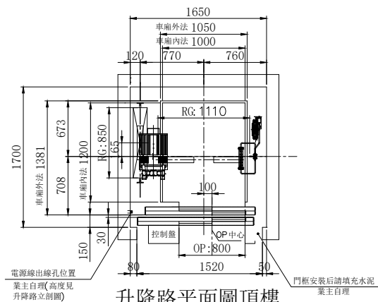
升降路平面圖頂樓
