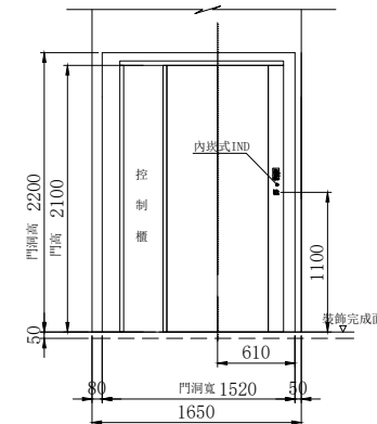
乘場門詳細圖頂樓
