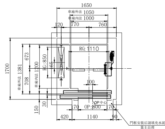
升降路平面圖其餘樓
