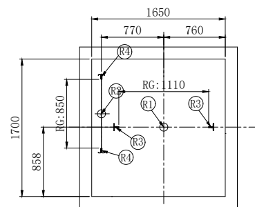
機坑平面圖
