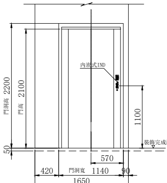
乘場門預詳細圖其餘樓
