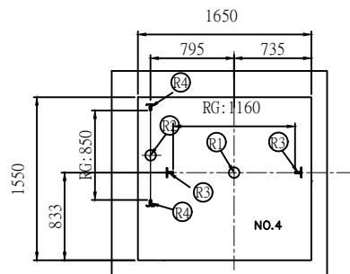
機坑平面圖
