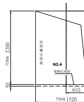
乘場門預留孔圖頂樓
