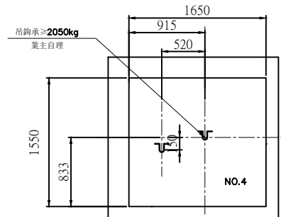
吊鉤位置示意圖
