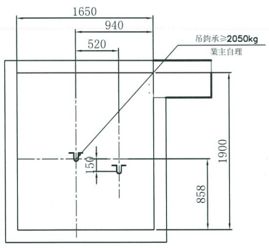
吊鉤位置示意圖
