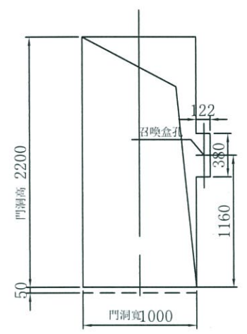
乘場門預留孔圖其餘樓
