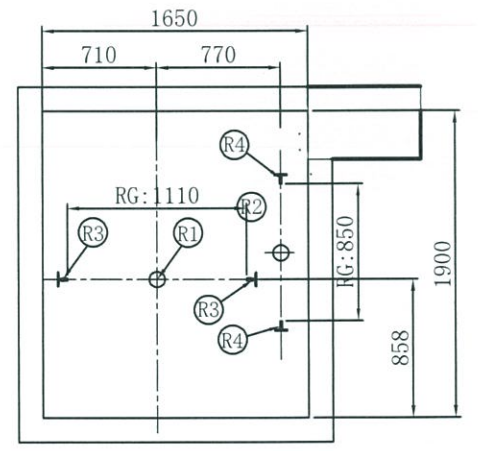
機坑平面圖
