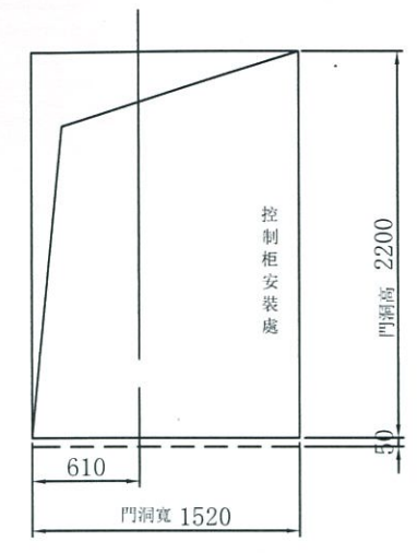
乘場門預留孔圖頂樓
