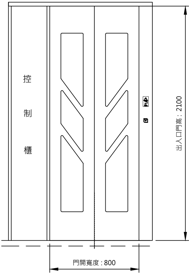
頂樓出入口詳細圖
