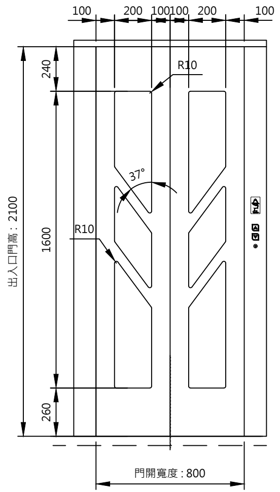
其他樓出入口詳細圖
